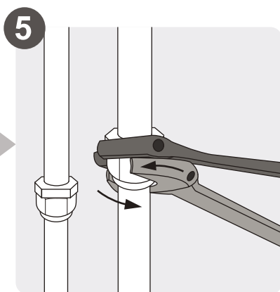
Свързване на тръбите
