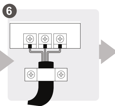
Свързване на кабелите
