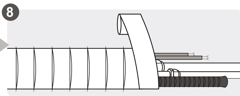
Бандажиране на пакета от тръби и кабели
