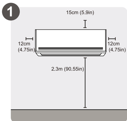
Избор на място за инсталиране
