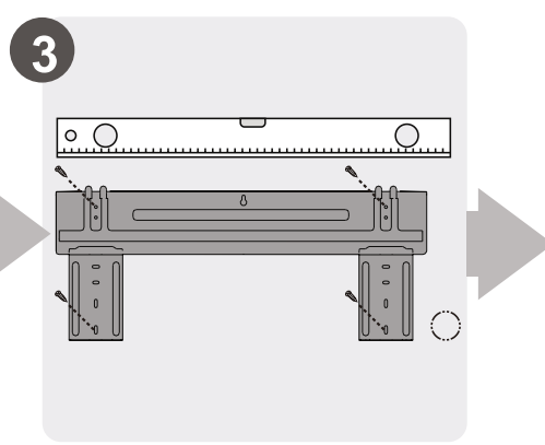
Инсталиране на монтажната основа
