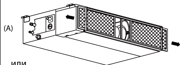
Модел със задна вентилация
